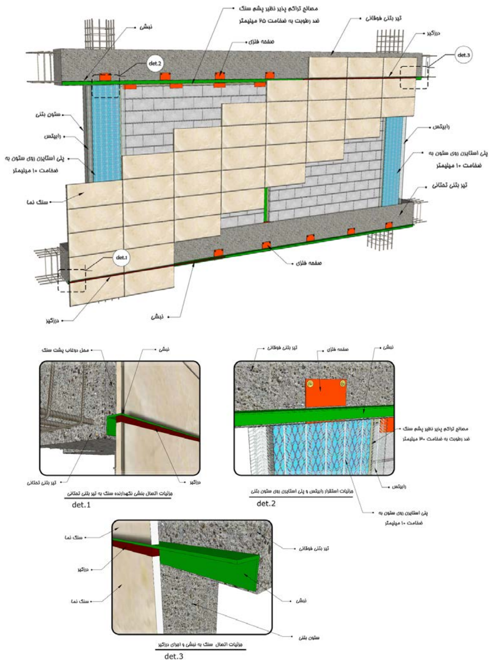
شکل پ-۲۵- نحوه اجرای نمای چسبانده شده در دیوارهای جداسازی شده
